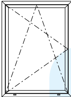
Abrir e Tombar 1 folha
